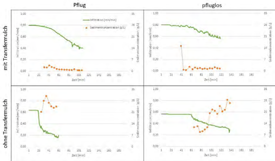
Abb. 1: Infiltrationskurve und Sedimentkonzentration des Abflusses der Beregnungsversuche auf Kartoffeln (© J. Schumann)
