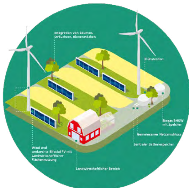
Abb. 1 Schematische Darstellung des Konzepts von vertikalen, bifacialen Solaranlagen zusammen mit Windenergie und Blühstreifen in der Landwirtschaft (© Fraunhofer IMW)
