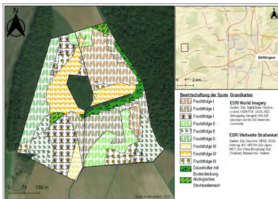
Abb. 1: Einteilung und Bewirtschaftung der homogenen Spots für eine der Beispielflächen nahe Göttingen. Die Einteilung der Spots erfolgte auf Datengrundlage der Bodenschätzungskarte (Maßstab 1:5.000 (LBEG 2020a)), der Bodenkarte (Maßstab 1:50.000 (LBEG 2020b)), des Digitalen Geländemodells (10-m-Raster (BKG 2019)) und einer Karte des Oberflächenabflussrisikos zum nächsten Gewässer (Geoinformationsdienst (GID) und Bayer Agrar Deutschland 2020). (© Julius Kühn-Institut)
