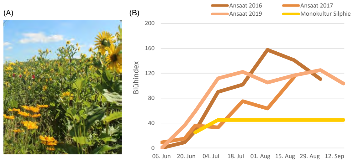
Abb. 1: (A) Vollblüte der Ansaat 2016; (B) Jahresverlauf 2019 des Blühindex der verschiedenen Ansaaten im Vergleich zu einer Monokultur Silphium perfoliatum (© Kornelia Marzini, LWG)
