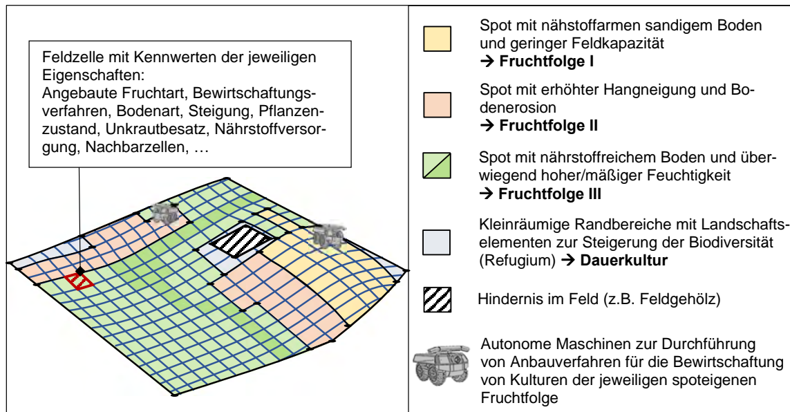
Abb. 1: Feld mit verschiedenen Spots gleicher Eigenschaften und Anbauverfahren. Einteilung der Spots nach Untersuchungen des JKI auf Basis verschiedener Geodaten und pflanzenbaulicher Kenntnisse. Maschinen führen in der Simulation Verfahren zur Bewirtschaftung der Spots und angebauten Kulturen durch.
