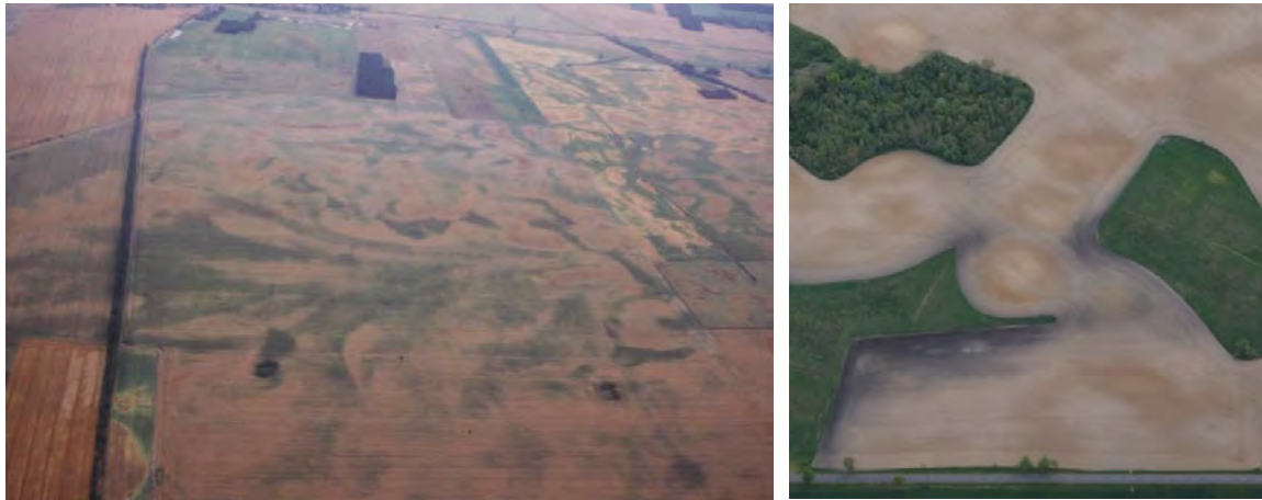
Abb. 2: Farb-Luftbild von Winterweizen am 07.07.1999 (links) und von fast unbedeckter Bodenoberfläche am 15.05.2020 (rechts) (© Dobers)
