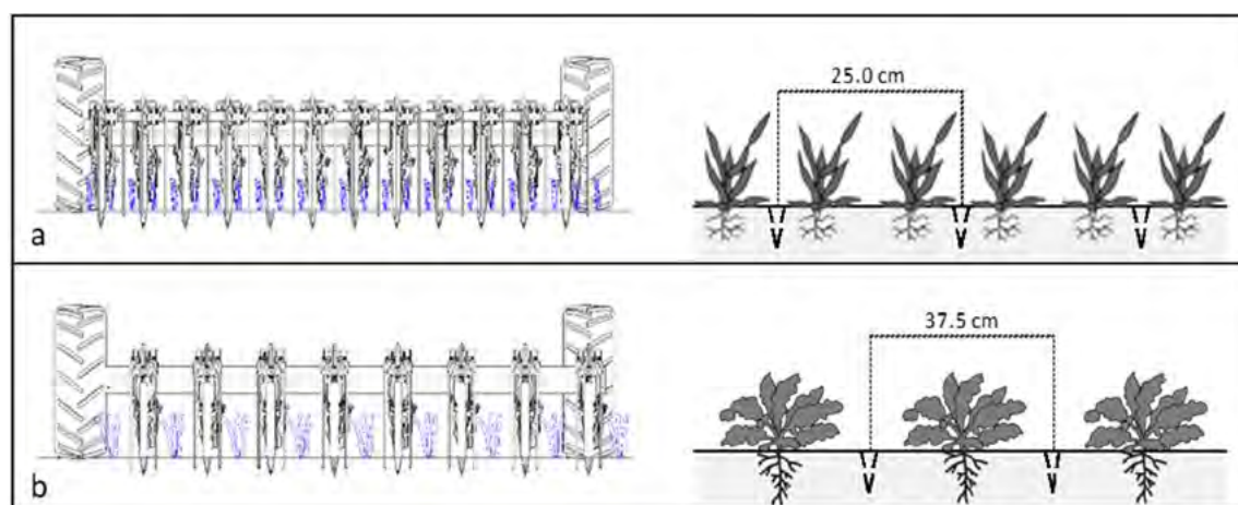
Abb. 1: Schematische Darstellung des Side-Dressing-Verfahrens in Getreide (a) und Raps (b)
