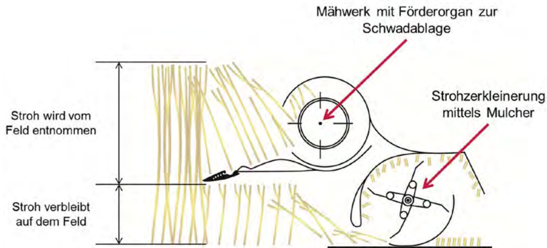
Abb. 1: Beispielhafte Darstellung Funktionsmuster „Kombi-Mulcher“ (Hanke et al. 2015)
